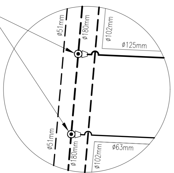
DETALLE "A"
